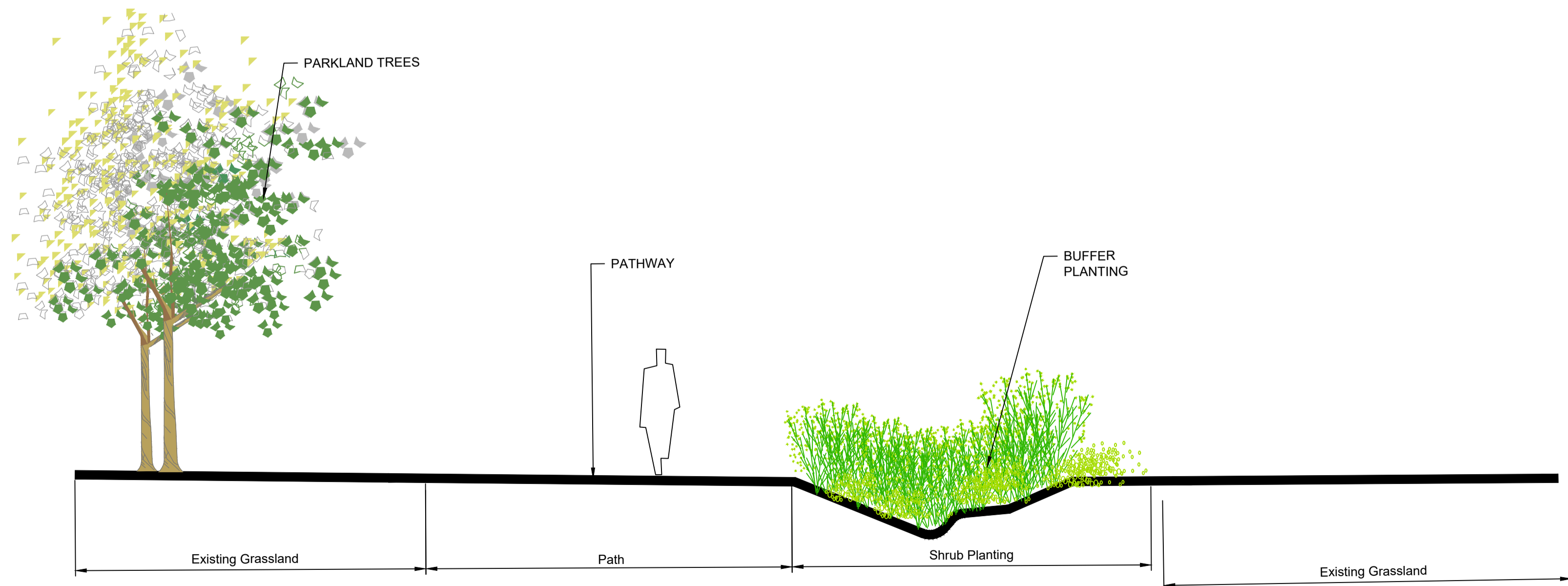
13 GREENWAY M-M SCALE: 1:50
